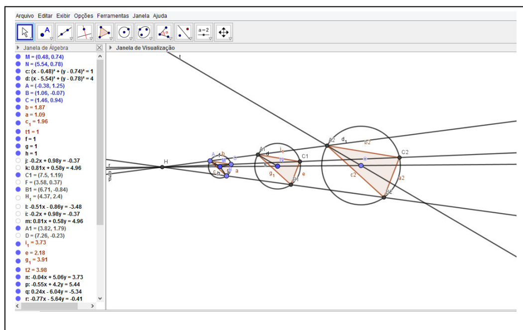
Figura 4: Triângulos inscritos homotéticos
