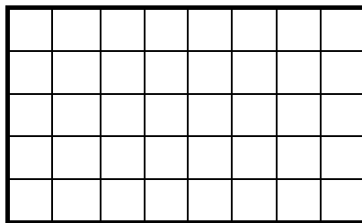
Fig. 4. Retângulo R , cujos lados medem 5 e 8, subdividido em 5 \times 8 = 40 quadrados unitários. Tem-se área de R = 8 \times 5 = 40 .
