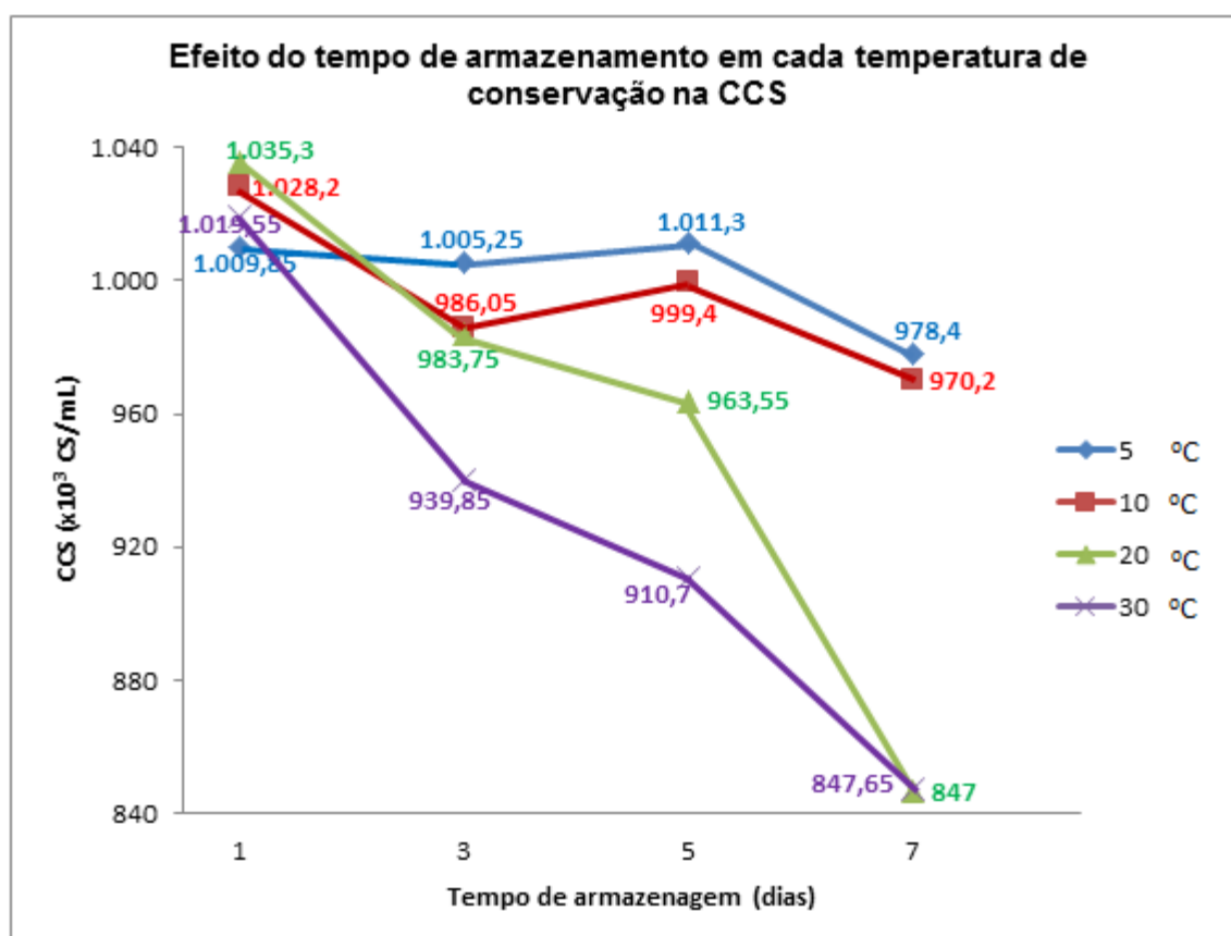
Gráfico 1 – Efeito do tempo de armazenamento em cada temperatura de conservação na CCS.
