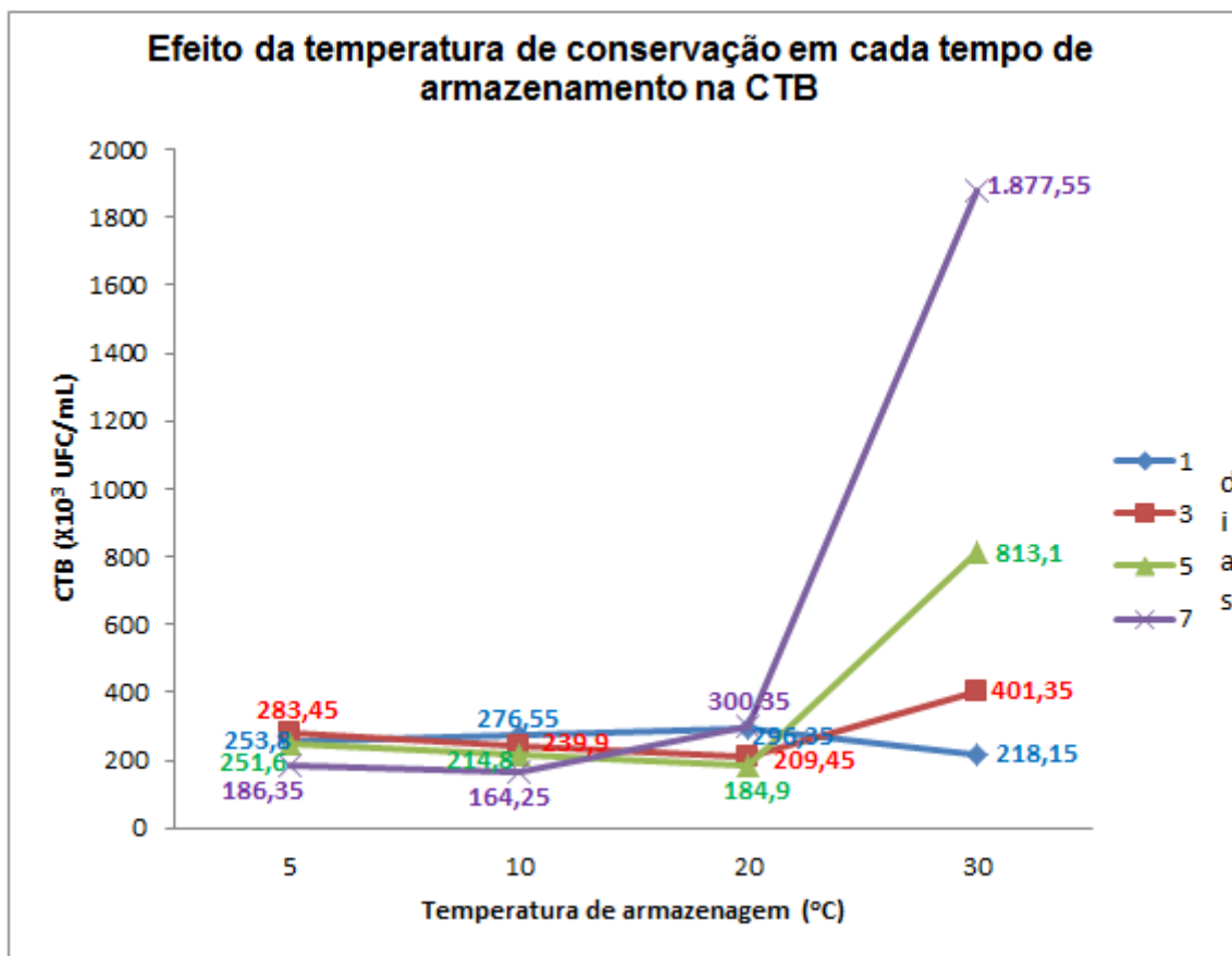
Gráfico 4 – Efeito da temperatura de conservação em cada tempo de armazenamento na CTB.
