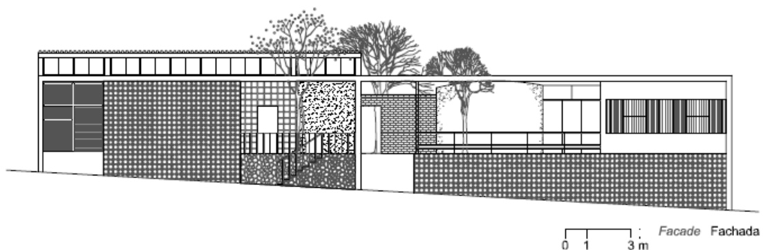
Figura 17. Projeto original das residências José de Castro e Wellington de Souza.
