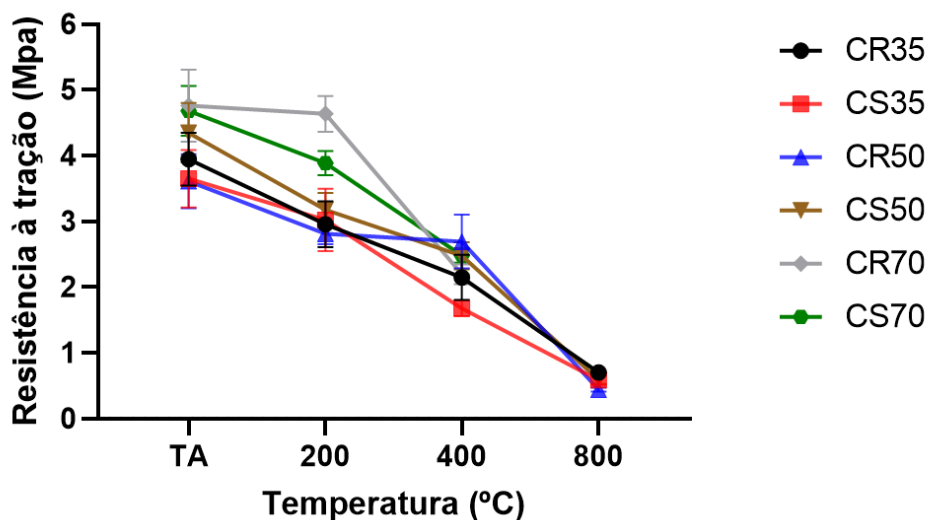
Gráfico 16 - Resistência a tração x Temperatura.
