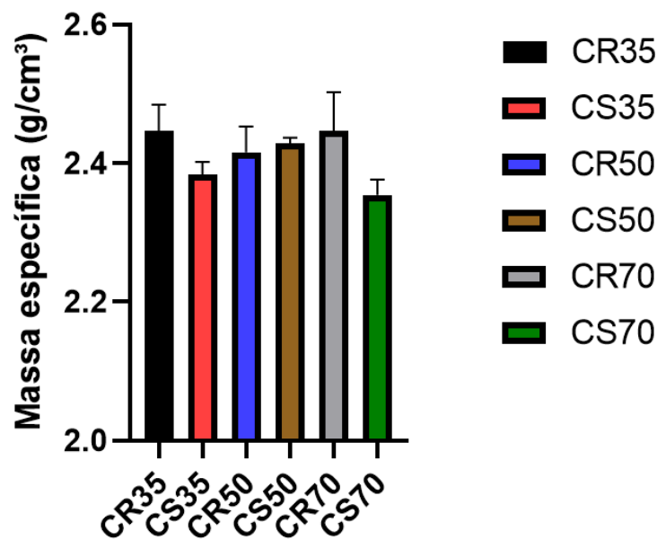
Gráfico 6 - Massa específica.
