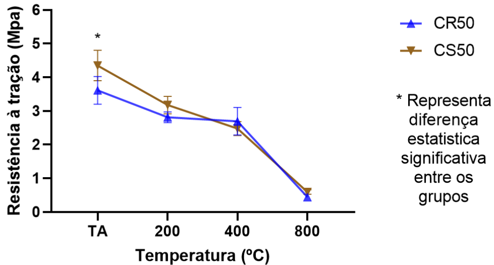
Gráfico 18 - Resistência à tração x Temperatura. Classe 50.
