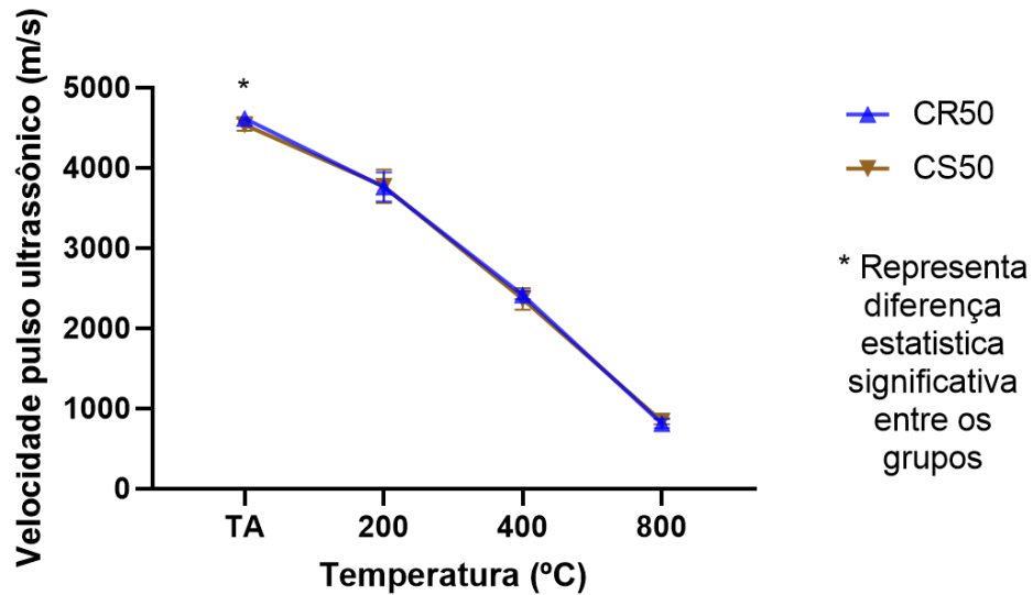
Gráfico 10 - Velocidade do pulso ultrassônico x Temperatura. Classe 50.
