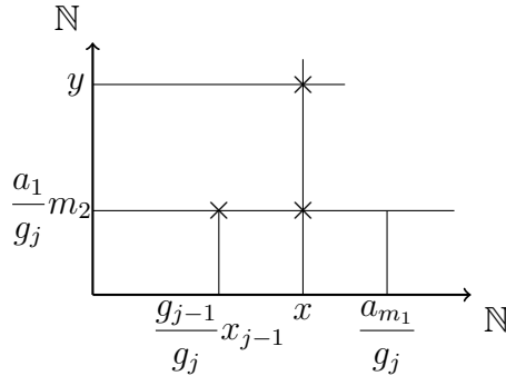
Figura 8 – Representação Gráfica da Afirmção 5.4
