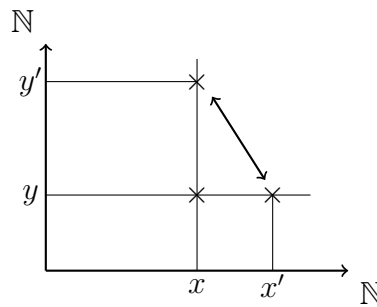
Figura 4 – Representação Gráfica da Propriedade B
