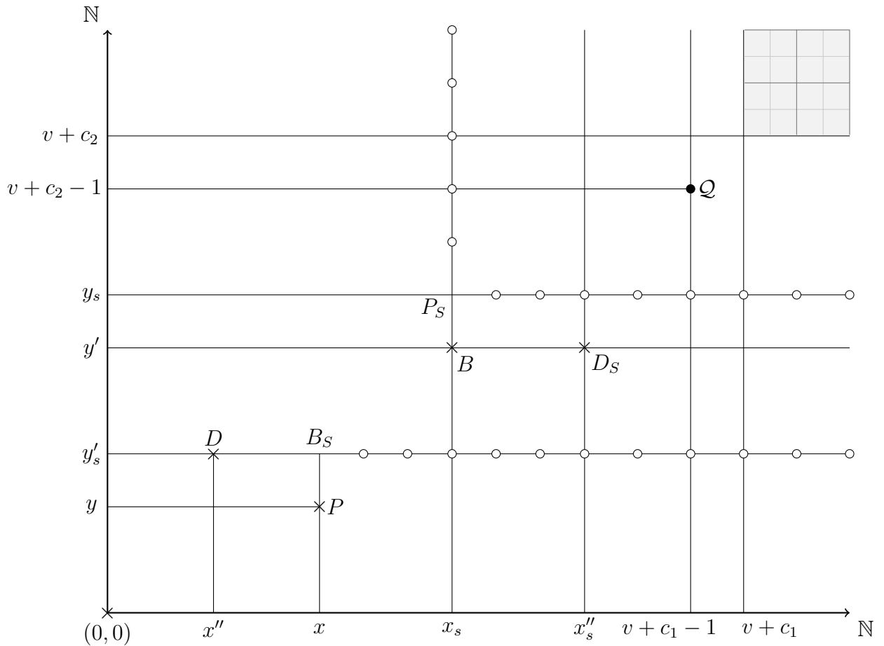
Figura 6 – Representação Gráfica do Teorema 5.3
