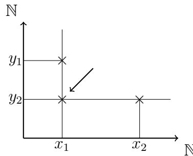
Figura 3 – Representação Gráfica da Propriedade A
