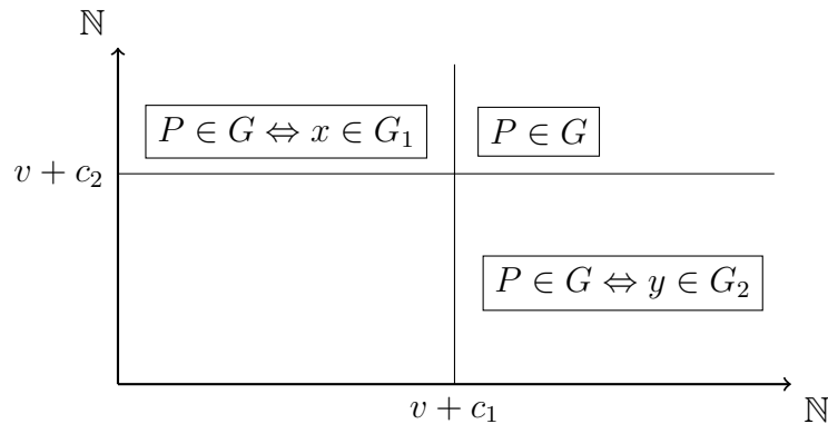
Figura 2 – Representação Gráfica do Teorema 4.2
