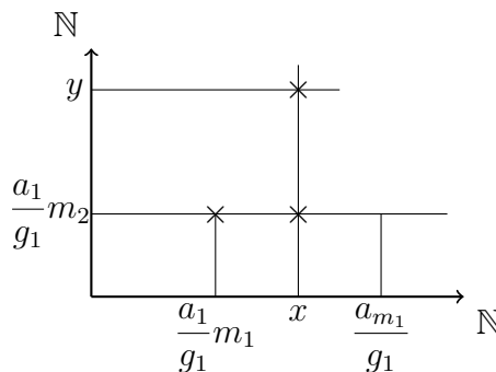
Figura 7 – Representação Gráfica da Afirmção 5.2
