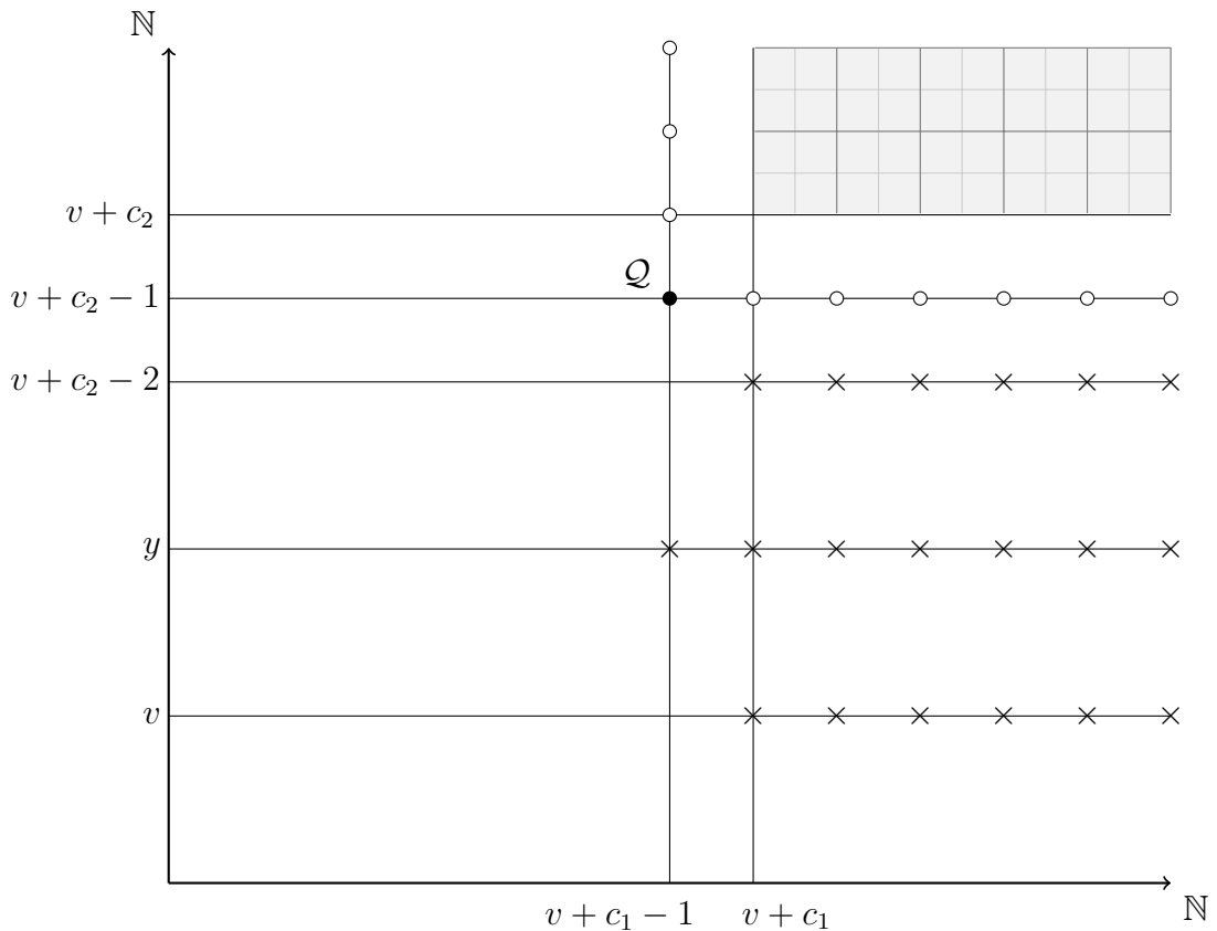
Figura 5 – Representação Gráfica do Caso 1 do Teorema 5.2
