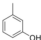
3-hidróxitolueno
