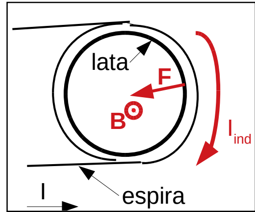
Vista Superior
