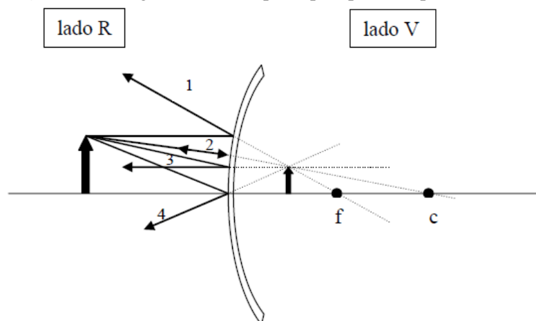
Figura 10 - Diagrama de raios principais para o espelho convexo
