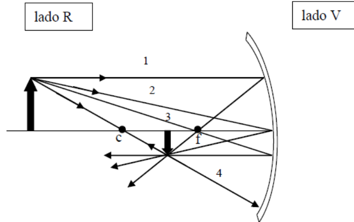
Figura 9 - Diagrama de raios principais para o espelho côncavo
