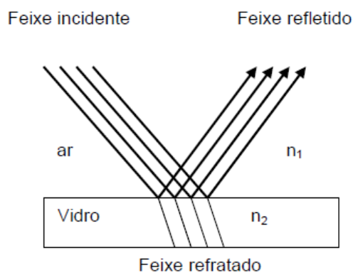
Figura 3 - Reflexão especular.
