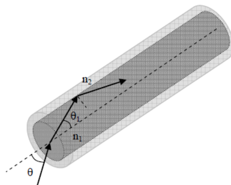
Figura 18 - Fibra óptica
