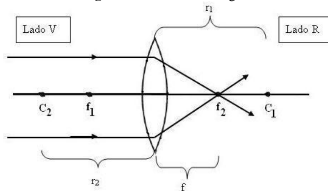
Figura 14 - Lente convergente
