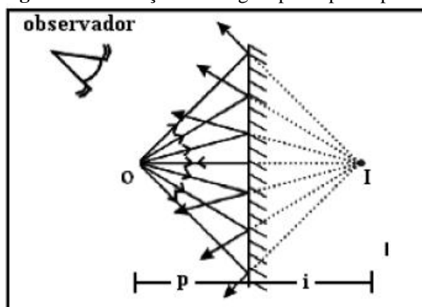
Figura 6 - Formação de imagem por espelho plano.
