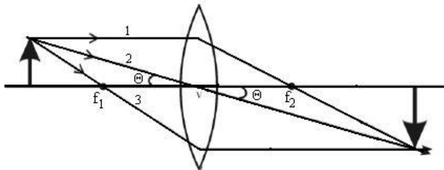
Figura 15 - Raios principais em uma lente convergente
