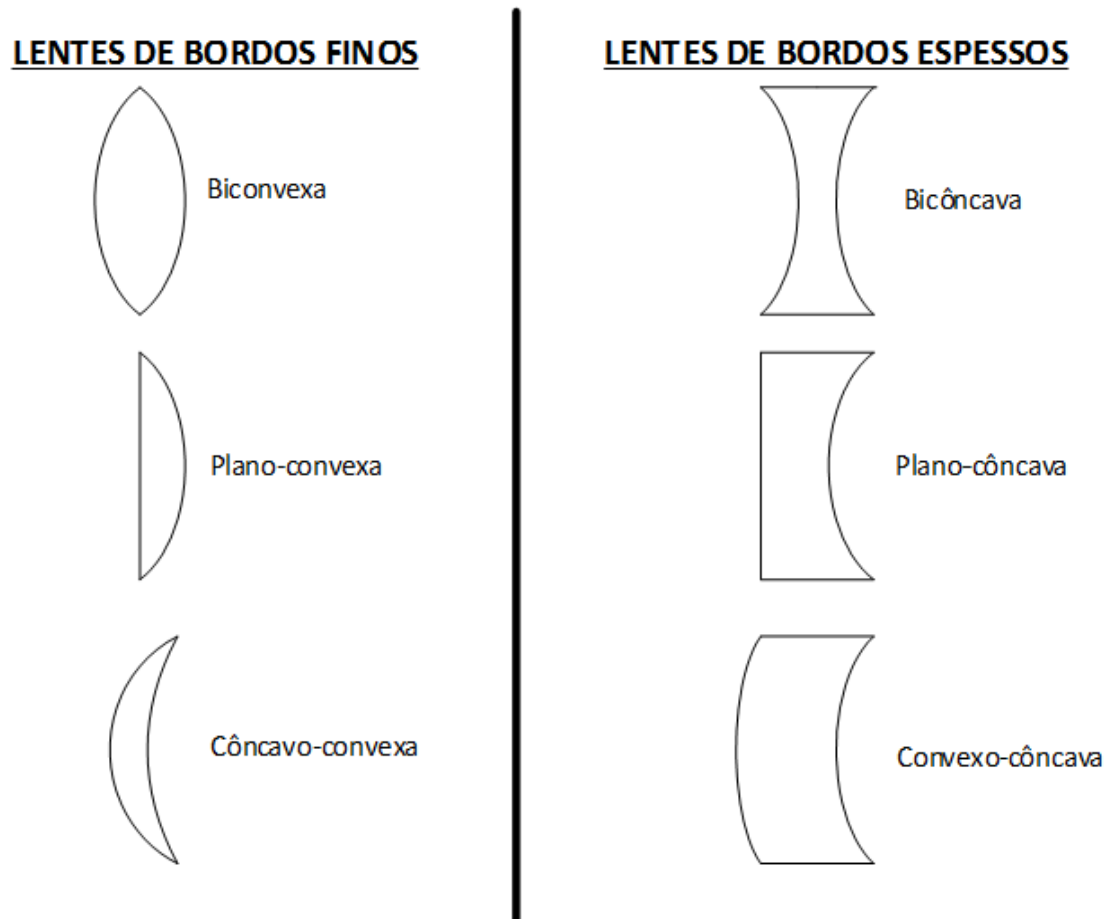
Figura 13 - Principais tipos de lentes
