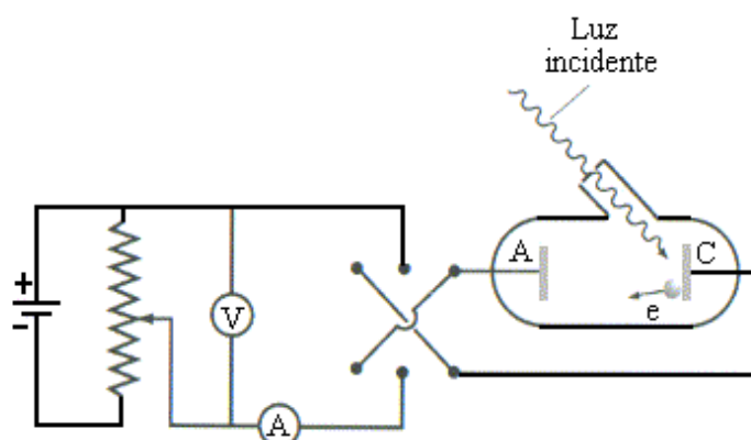
Figura 2 - Esquema do aparelho básico para o estudo do efeito fotoelétrico.
