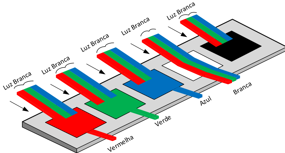
Figura 21 - Absorção e reflexão da luz por diferentes pigmentos
