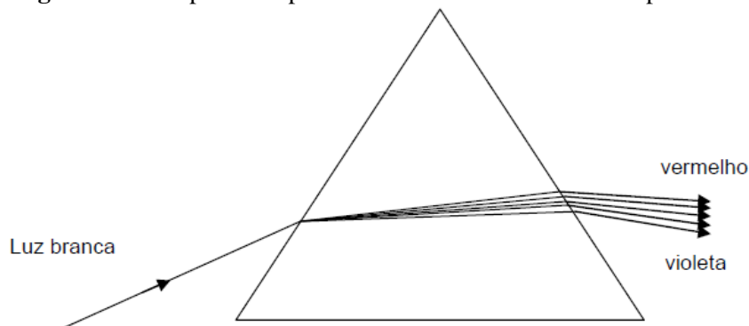
Figura 20 - Um prisma separando a luz branca em suas componentes
