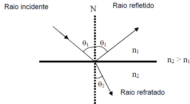
Figura 12 - Reflexão e refração de um raio de luz incidente em uma superfície plana
