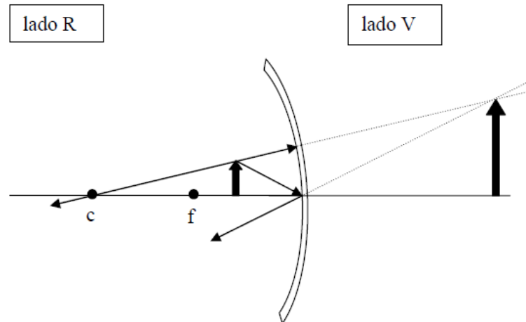
Figura 11 - Formação de imagem por espelho côncavo
