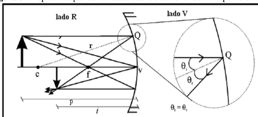
Figura 8 - Representação da validade das leis da reflexão no espelho esférico
