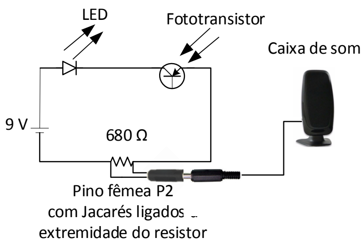
Figura 21 - Esquema de montagem do aparato experimental
