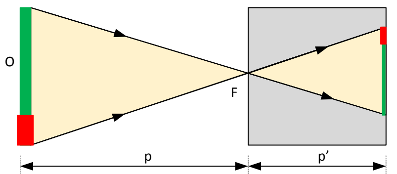
Figura 11 - Relações trigonométricas presentes na câmara escura de orifício.
