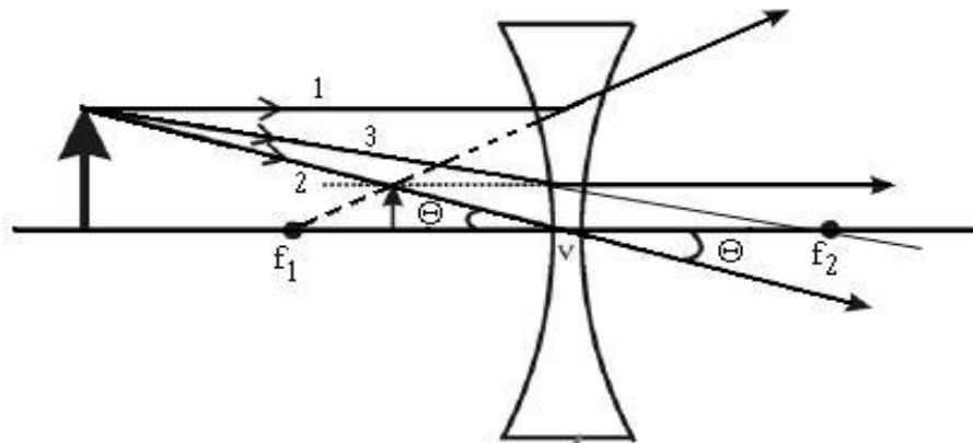
Figura 16 - Raios principais em uma lente divergente
