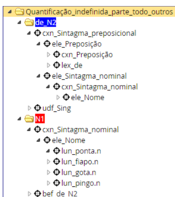
Figura 46: Restrições aplicadas à Quantificação_indefinida_parte_todo_outros
