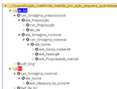
Figura 44: Restrições aplicadas à Quantificação_indefinida_Medida_por_ação_pequena_quantidade
