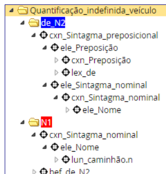
Figura 48: Restrições aplicadas à Quantificação_indefinida_veículo
