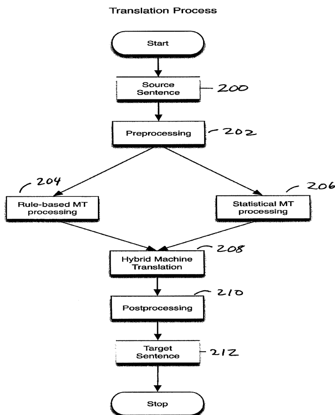
Figura 8: Processo de tradução híbrida do Google Translate
