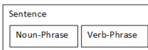
Figura 15: Construção Sujeito-Predicado
