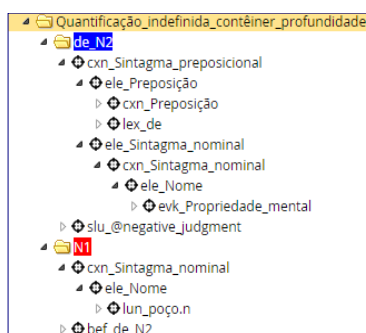
Figura 38: Restrições aplicadas à Quantificação_indefinida_contêiner_profundidade
