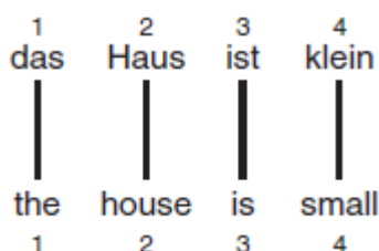
Figura 4: Alinhamento de cada palavra do alemão para o inglês
