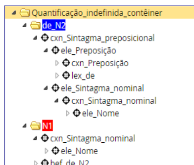
Figura 37: Restrições aplicadas à Quantificação_indefinida_contêiner
