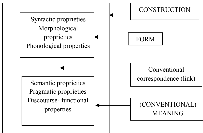
Figura 28: Estrutura simbólica da construção
