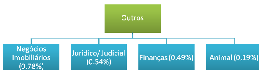
Figura 44: Detalhamento das temáticas sob o rótulo de “Outros”
