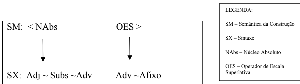
Figura 35: A Construção Superlativa Genérica (Sintética ~ Analítica) de Estados Absolutos
