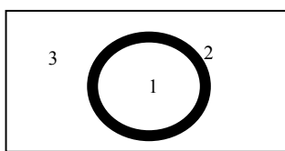
Figura 41: Diagrama do esquema imagético do container
