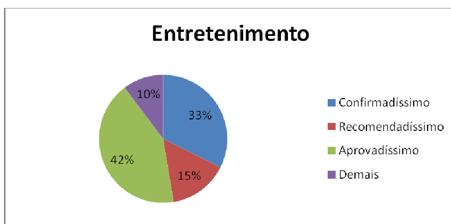
Figura 45: Gráfico - Temática Entretenimento e os types que a articulam
