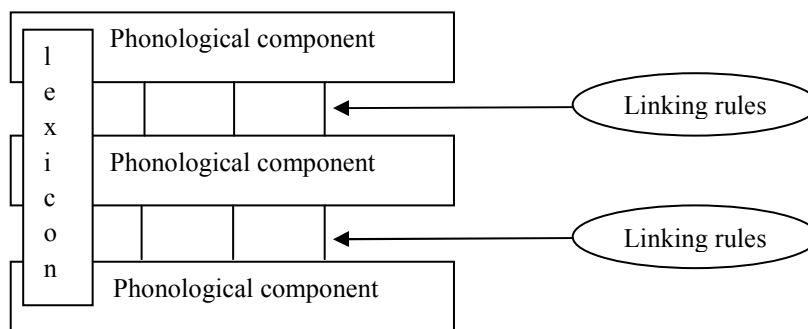
Figura 27: Modelo de organização do conhecimento gramatical das teorias sintáticas
