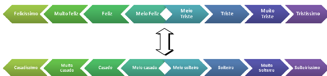
Figura 37: Relação entre a escala harmônica e a desencontrada
