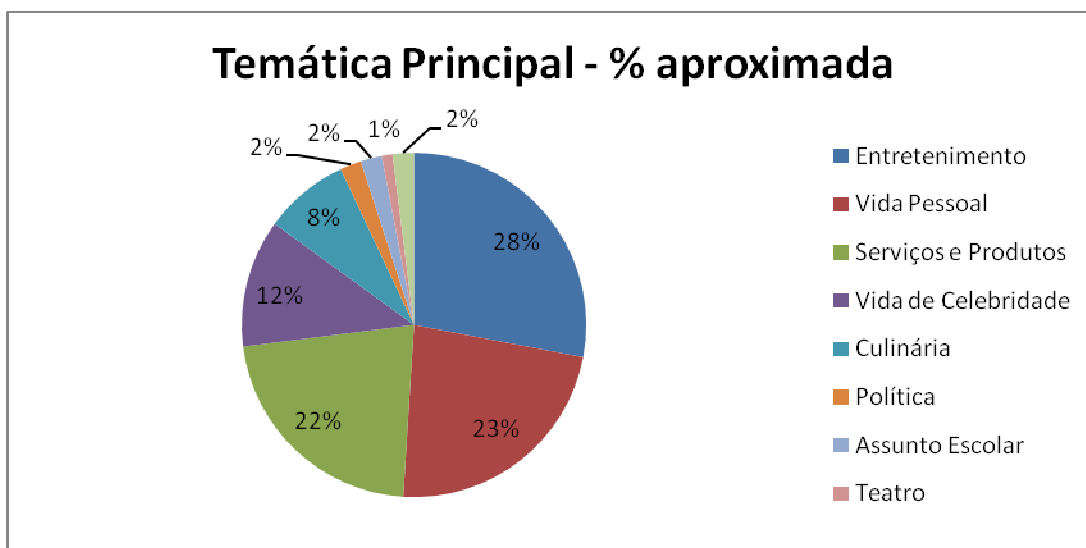
Figura 43: Gráfico – Temática Principal e Porcentagem aproximada
