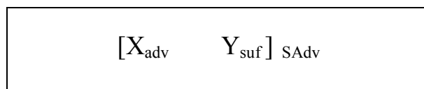
Figura 40: Padrão Formal das CSSEA com núcleo adverbial
