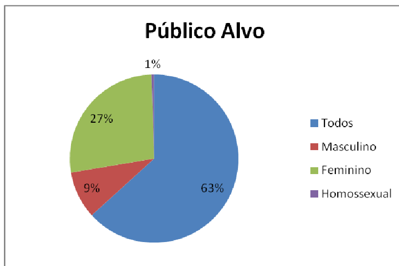
Figura 48 Gráfico da tendência em relação ao público alvo
