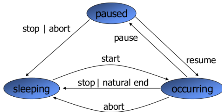
Figura 2.3: Máquina de estados de eventos (COSTA, 2010)
