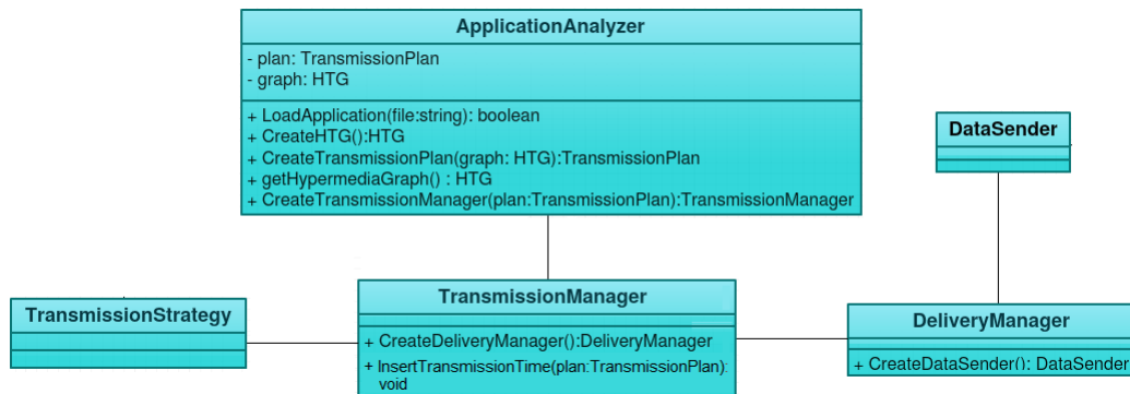
Figura 4.3: Elementos responsáveis pelo gerenciamento da transmissão
