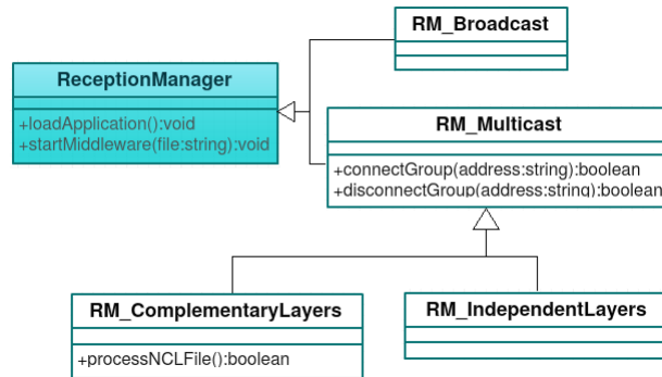
Figura 5.3: Instanciação do componente ReceptionManager
