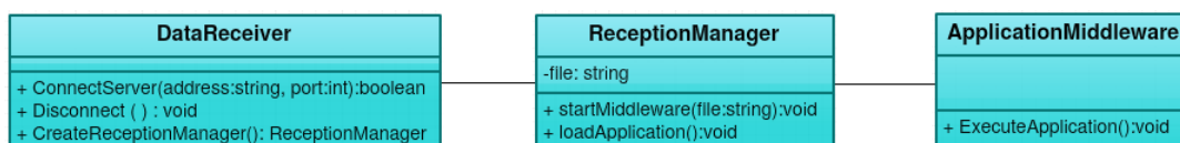
Figura 4.4: Elementos responsáveis pela recepção do conteúdo
