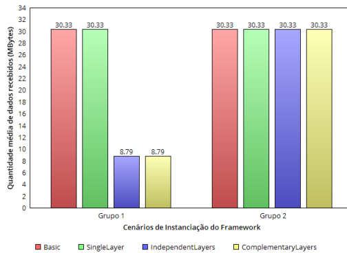
Figura 6.5: Quantidade de dados recebidos, por grupo de usuários, para aplicação 2
