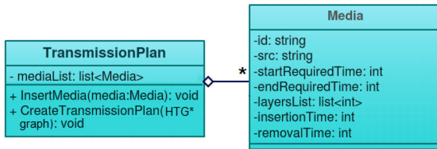
Figura 4.2: Definição do plano de transmissão
