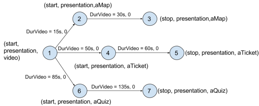
Figura 2.5: HTG para o trecho de aplicação apresentado na Figura 2.4
