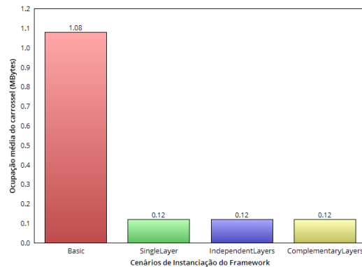
Figura 6.3: Ocupação média do carrossel para aplicação 1
