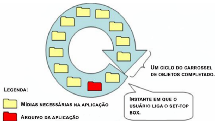
Figura 2.6: Carrossel de objetos contendo objetos de mídia de uma aplicação
