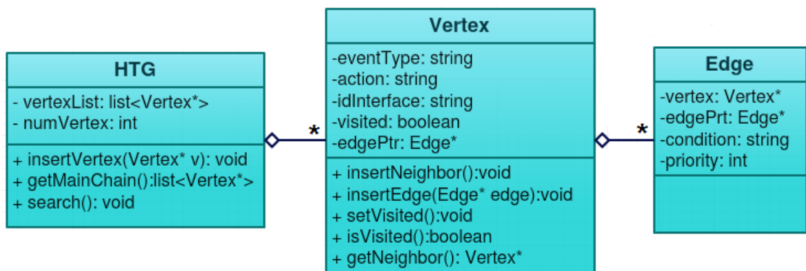
Figura 4.1: Definição do grafo temporal hiperímídia
