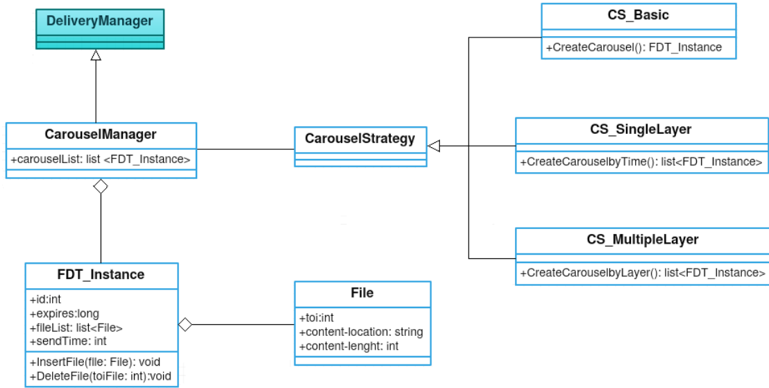
Figura 5.2: Instanciação do componente DeliveryManager
