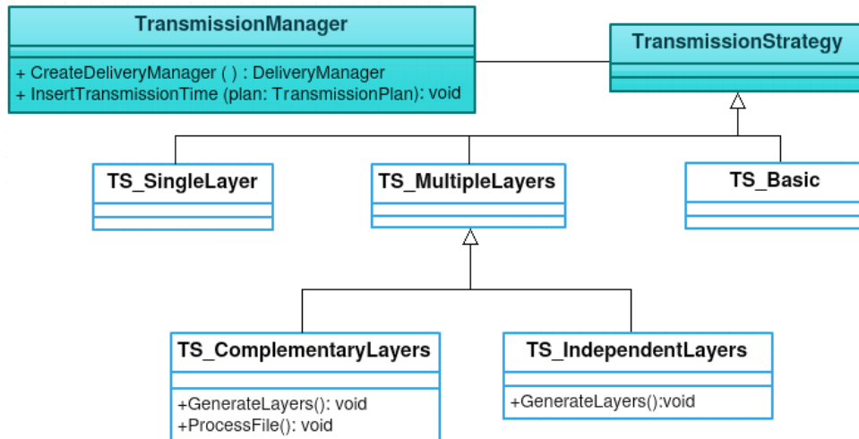
Figura 5.1: Instanciação do componente TransmissionStrategy
