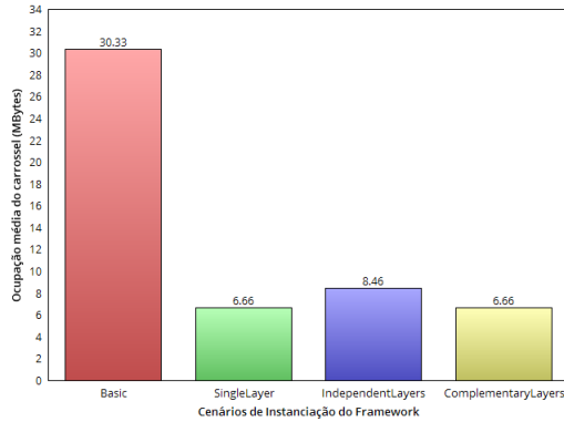
Figura 6.4: Ocupação média do carrossel para aplicação 2
