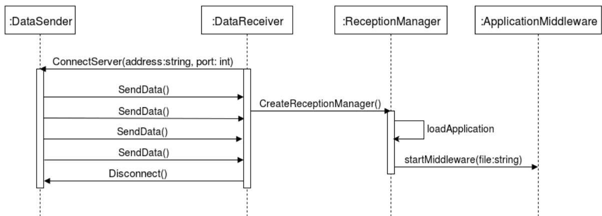
Figura 4.5: Diagrama de sequência do processo de recepção do conteúdo
