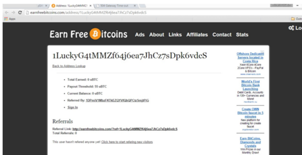
Figura 42 – Identificando usuários 3.
