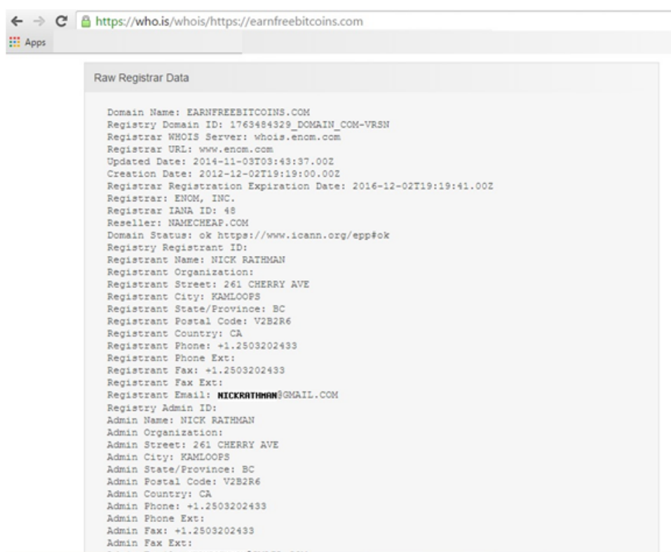
Figura 43 – Identificando usuários 4.
