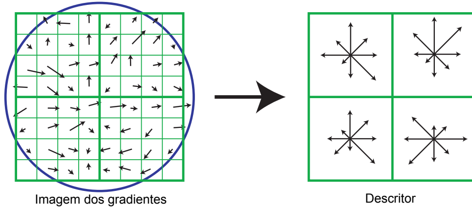
Figura 2.8: Exemplo do cálculo do descritor HOG (LOWE, 2004).
