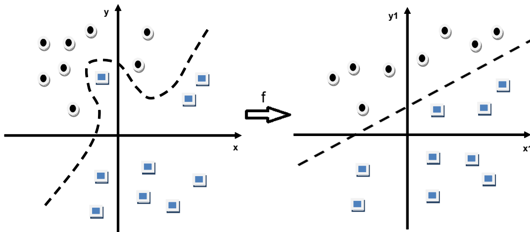
Figura 2.10: Os vetores são levados a uma dimensão maior por meio de uma função kernel f para que seja possível encontrar um hiperplano separador.
