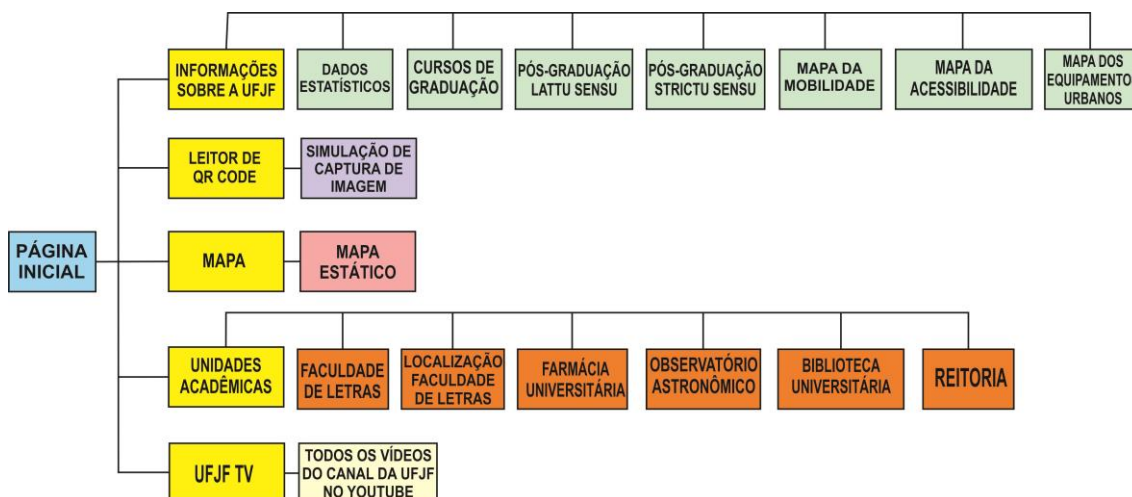
Figura 42 – Fluxograma do protótipo Alfa versão 9.0 do aplicativo “No Campus”.
