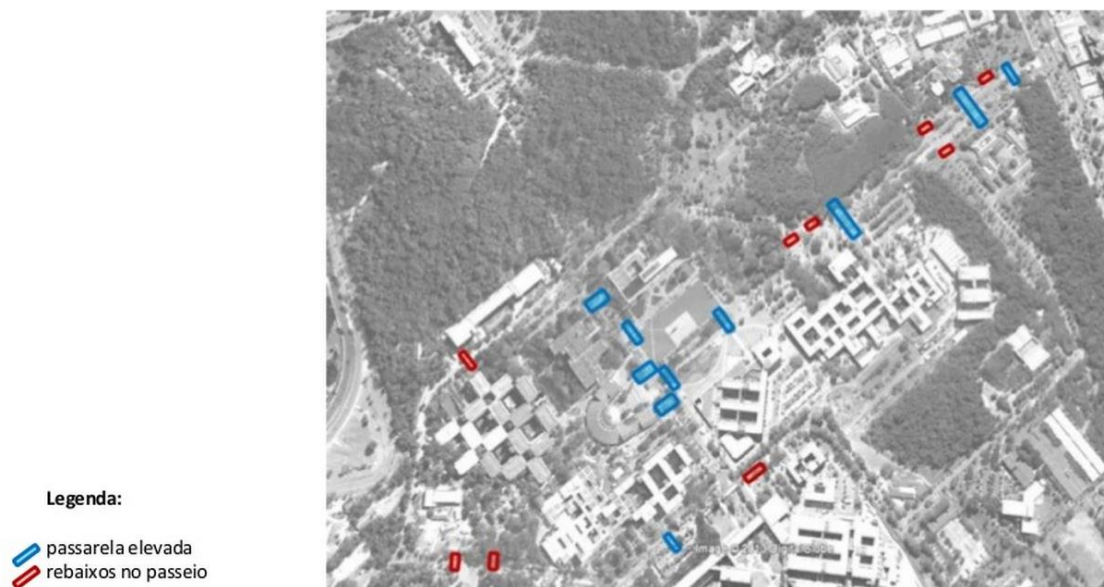
Figura 12 – Mapa geral da área central em estudo com proposições de passarela elevada e de rebaixos no passeio no campus da UFMG, na Pampulha – Belo Horizonte.
